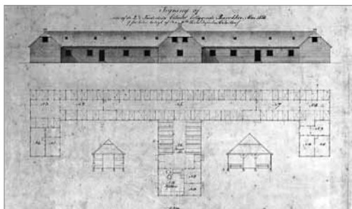
En-etages barak opført i Fredericia 1849. To nøjagtig tilsvarende blev opført i Ulkebøl. Ingeniørkorpsets historiske tegningsarkiv, Rigsarkivet
