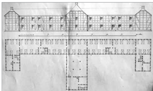
To-etages barak af hvilke der opførtes to i Ulkebøl. Man ser her bindingsværkskonstruktionen som ikke var synlig i virkeligheden, da konstruktionen var beklædt med brædder. Ingeniørkorpsets feltarkiv, Rigsarkivet
